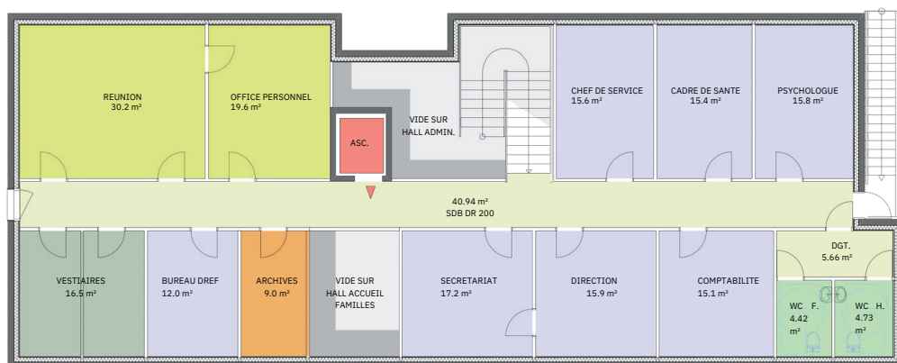
ACCUEIL DE JOUR ET ADMINISTRATION PLANS ADMINISTRATION - ETAGE
